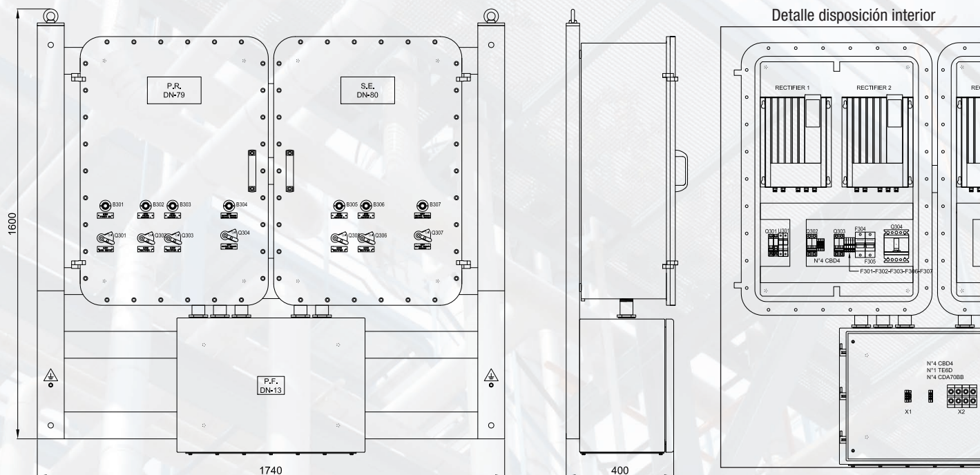
Ejemplo de panel de control con sistema de bastidor a pared.
