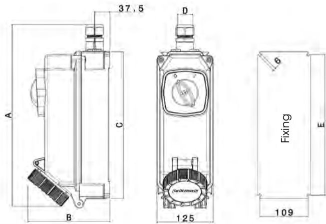
Sockets
